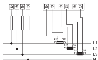
4 hilos / 4 wires
