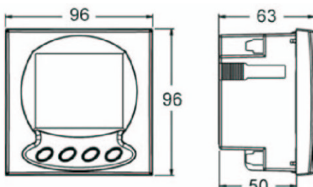
Dimensiones de la caja Case dimensions
